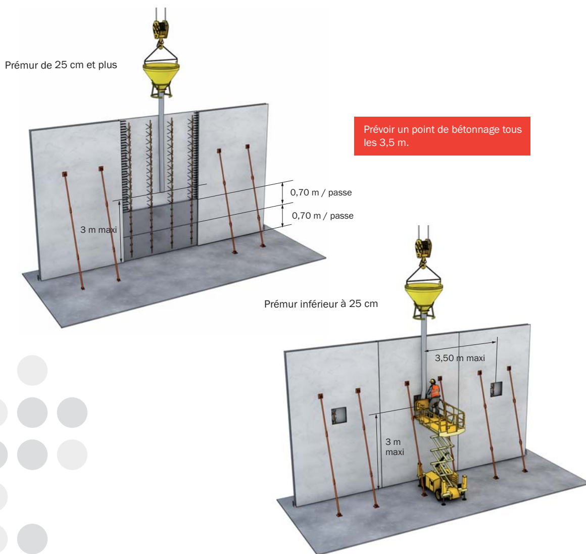
Hauteurs de chutes de béton
