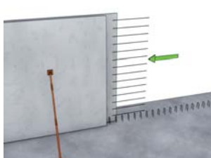
2 Ripage des armatures de liaison dans le prémur 1
